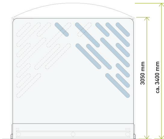
SEITENANSICHT: Fenster Rechts/Links
