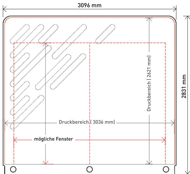
DRUCKPLAN-SCHEMA: Wand Innen
