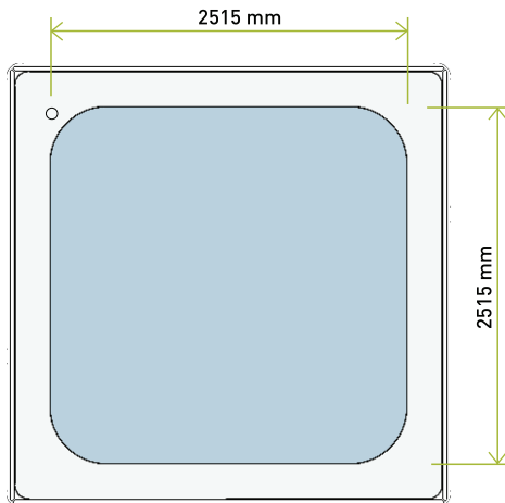
DRAUFSICHT: Pneumatische Dachmembrane transparent
