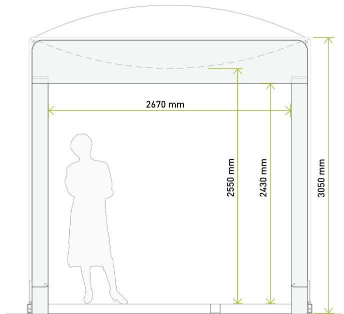
VORDERANSICHT: Geöffnet
