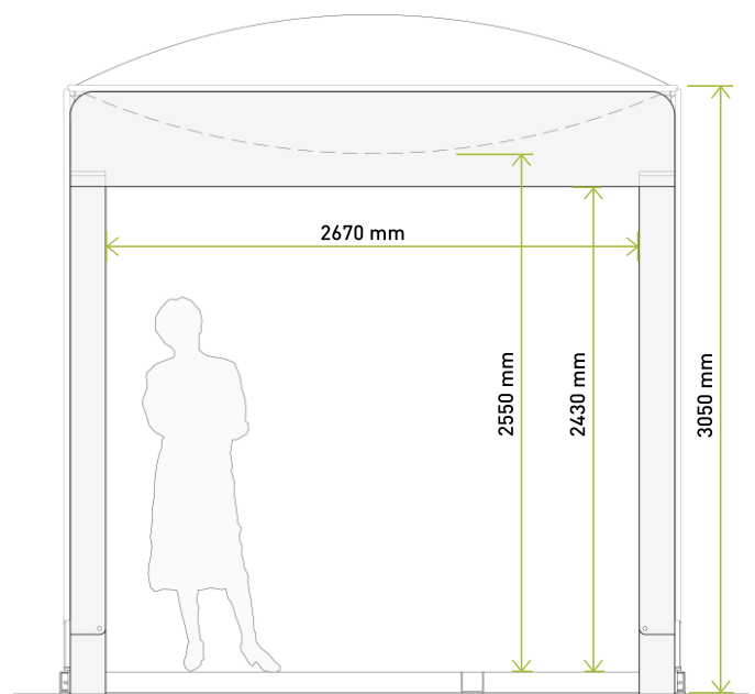
VORDERANSICHT: Geöffnet
