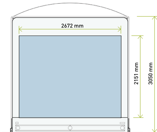
SEITENANSICHT: Zentral-Fenster
