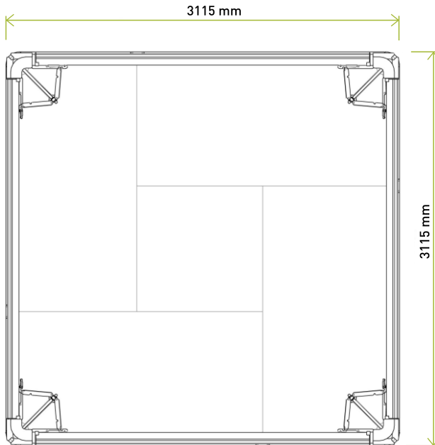
DRAUFSICHT: STRUKTUR
