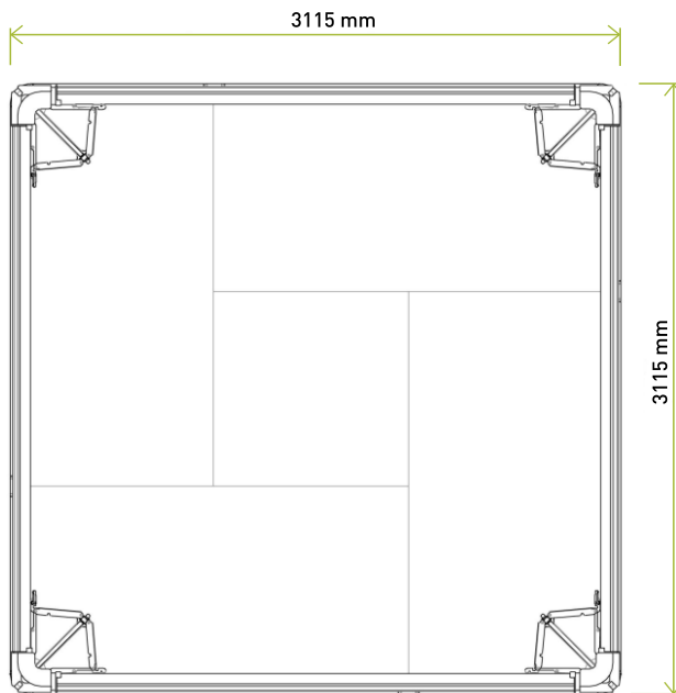
DRAUFSICHT: STRUKTUR
