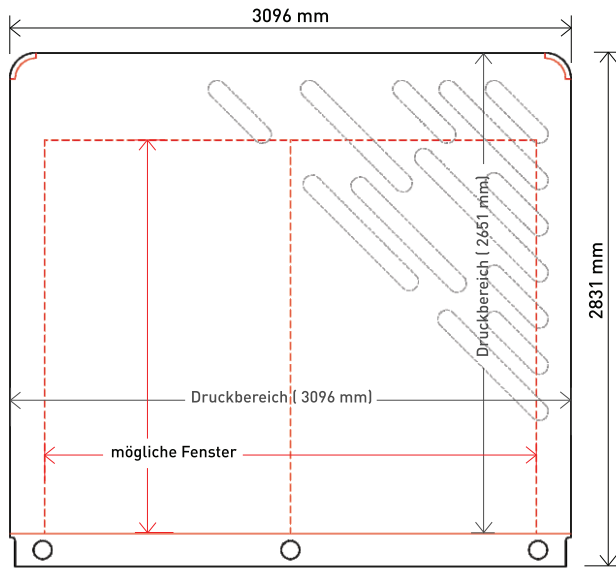
DRUCKPLAN-SCHEMA: Wand Außen
