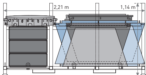
LÄNGSSCHNITT: Bodenrunge
